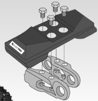
CADENA SOBRE TACO DE GOMA
