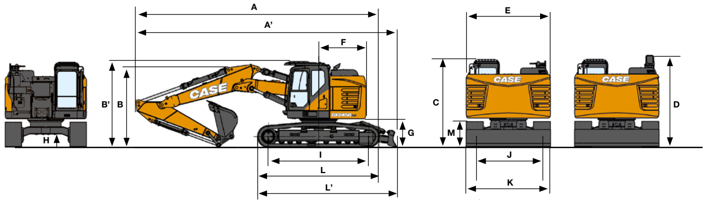
CX245D SR TRIPLE ARTICULACION (SIN HOJA)
