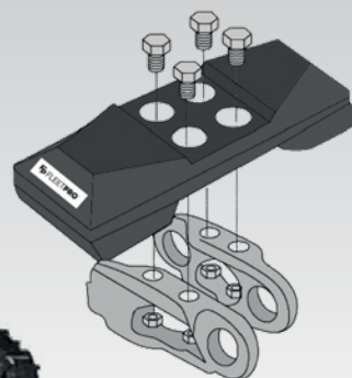
ЦЕПНЫЕ НАКЛАДКИ
