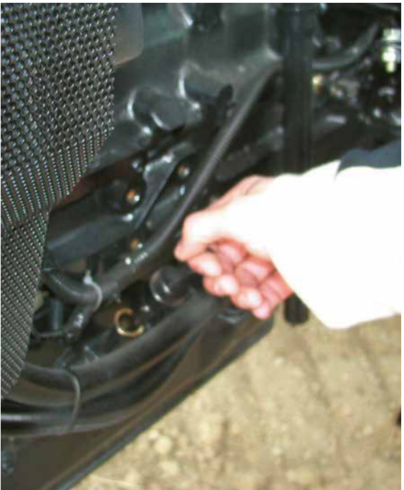
Inspección del aceite del motor sin levantar el capó.
