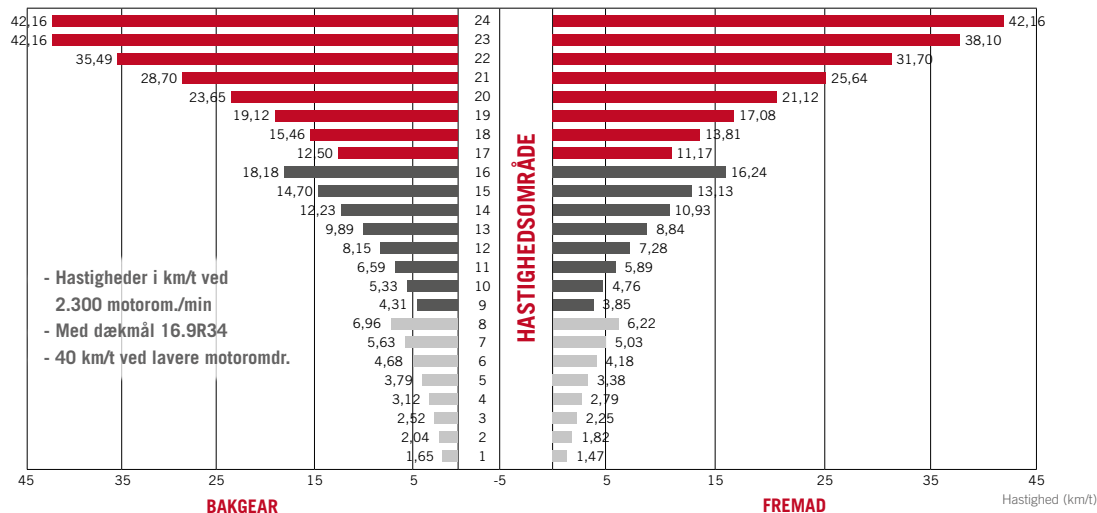
Hastighedsdiagram 24x24 transmission Hi Lo 40 km/t
