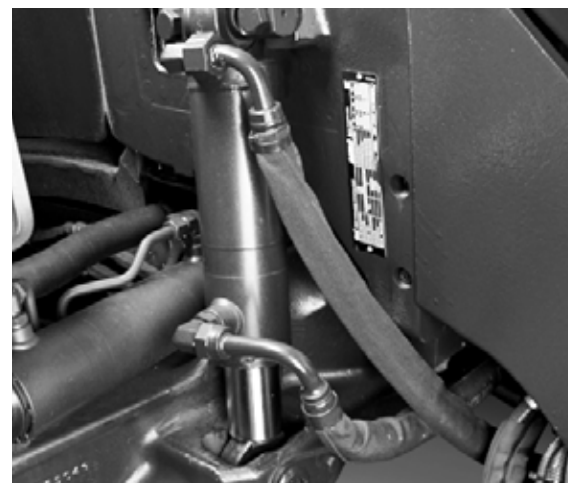
Full stabilitet, körning och full kraft mot marken tack vare framaxelfjädringen.
