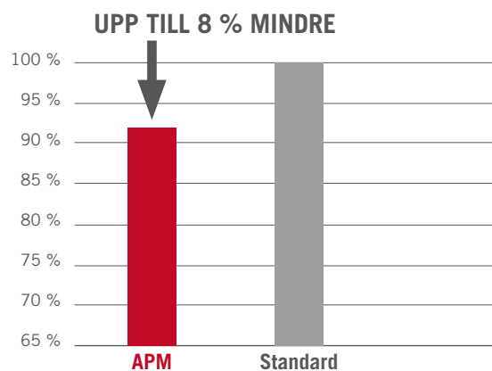
Auto Road: minskad bränsleförbrukning genom att använda detta läge
